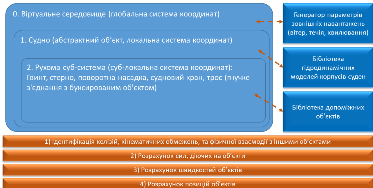
Рисунок 9 - Схема програмної реалізації групи суден в середовищі симулятора методами об'єктно орієнтованого програмування
