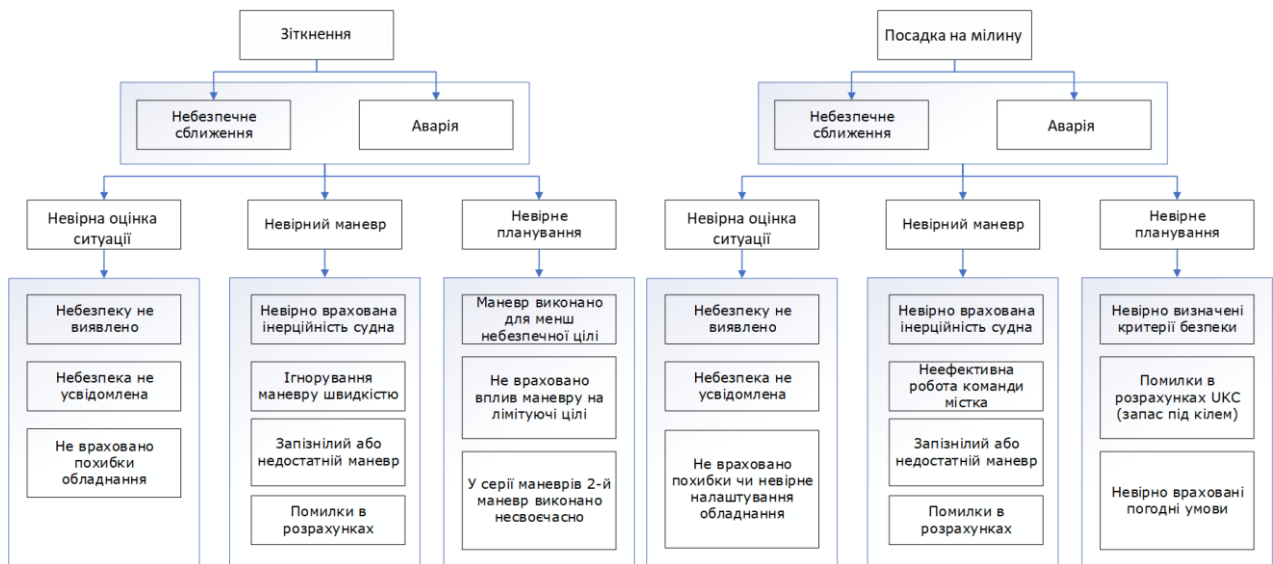
Рисунок 2 - Структура помилок, які можуть призвести до зіткнення (ліворуч) чи посадки на міліну (праворуч).
