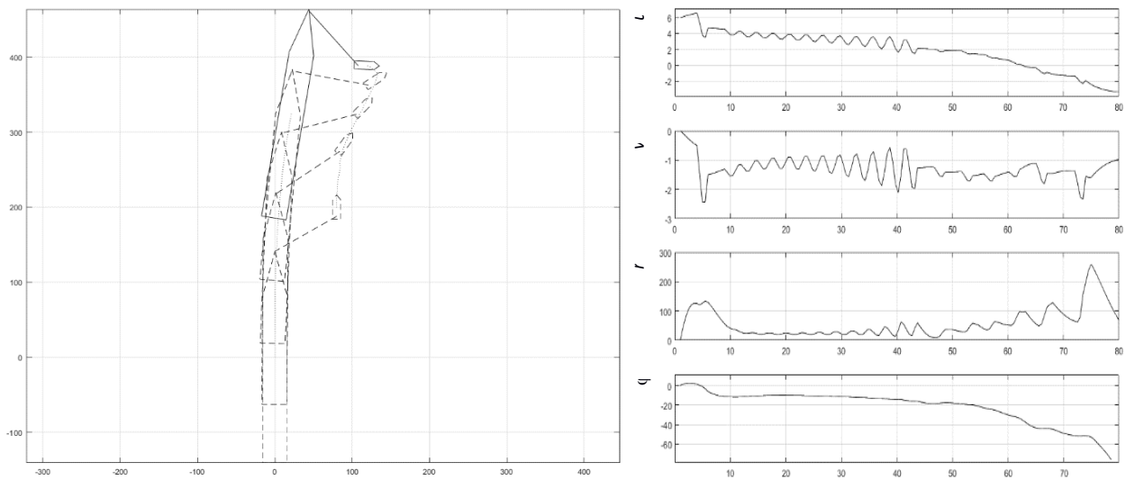
Рисунок 14 - Моделювання ситуації «гіртинг». Режим «stern-to-bow», швидкість – 6 вузлів
