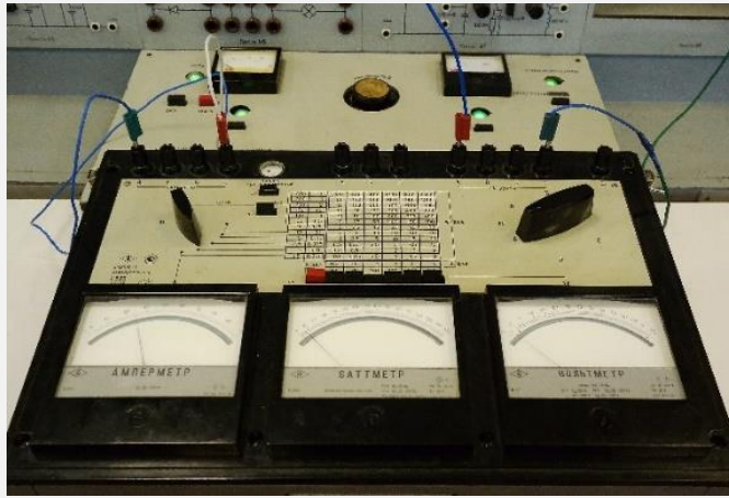
Рис.3 – Комплект вимірювальний К-505 (8 шт.)
